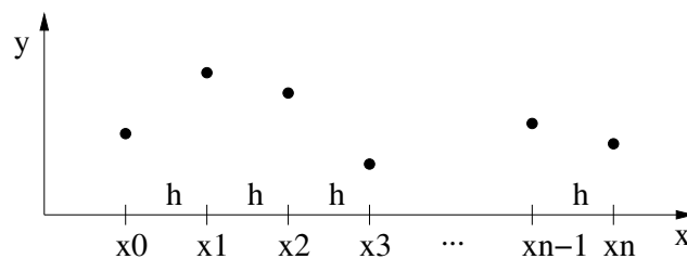
Abbildung 2: Visualisierung der äquidistanten Stützstellen x_i .
