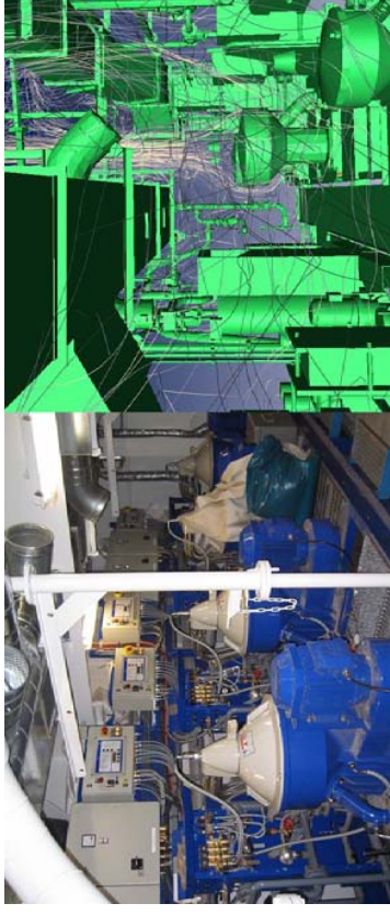
Abbildung 1: LES Lattice Boltzmann Simulation der turbulenten konvektiven Luftströmung in einem Separatorenraum (freie Konvektion, Ra \approx 10^{10} ), 295.899 Facetten, 24 Millionen Freiheitsgrade (van Treec et al. 2007)
