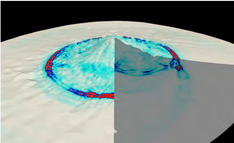
Abbildung 2: Momentaufnahme des seismischen Wellenfeldes am Vulkan Merapi: Reflexionen und Refraktionen an der Topographie und internen Schichten erhöhen dessen Komplexität.
