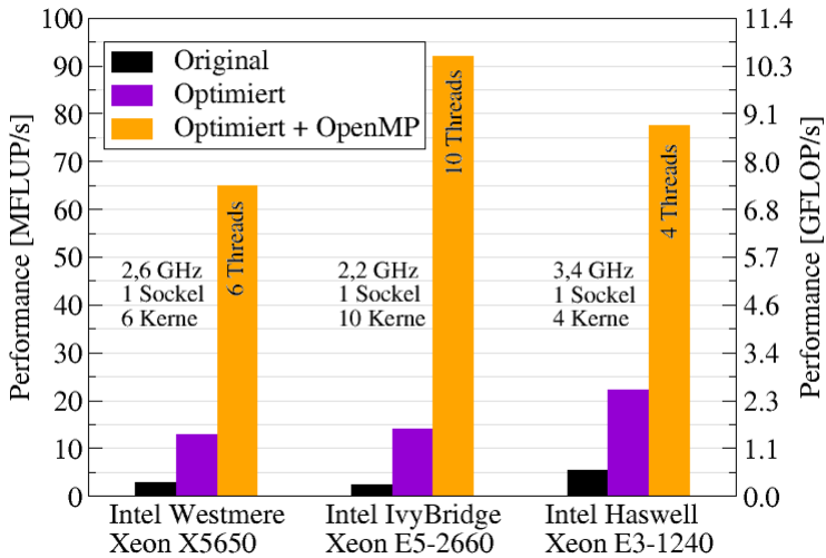
Abbildung 4: Performance des 2D-Lattice-Boltzmann-Strömungslösers für ein Gebiet von 100 \times 100 Knoten vor und nach der Code-Optimierung auf verschiedenen Prozessoren.
