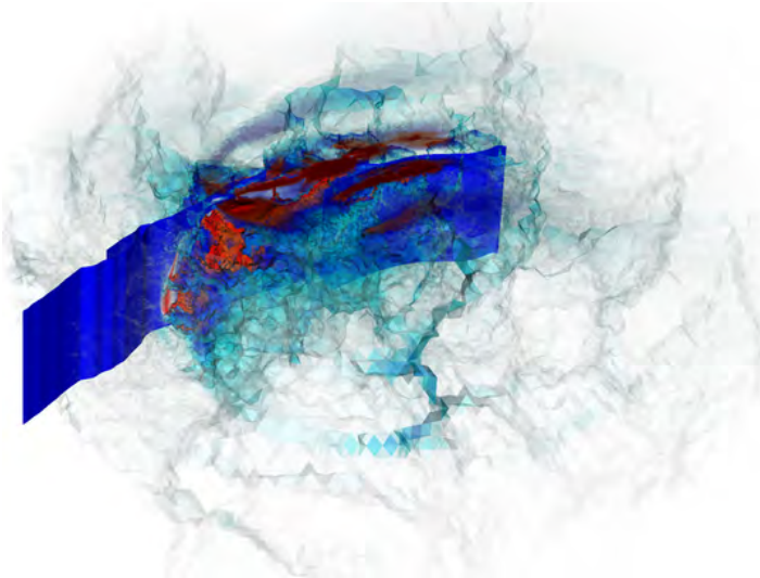
Abbildung 2: Visualisierung der Bruchfläche (dunkelblau), der sich ausbreitenden Erdbebenwellen (hellblau) sowie der resultierenden Bodenbewegung an der Erdoberfläche (rot) während des simulierten Erdbebens (Landers 1992).
