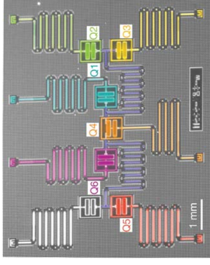
Abbildung 2: Ein von IBM entwickelter Quantenprozessor [2]. Die Komponenten sind in Falschfarben dargestellt. Einzelne superconducting qubits (Schwingkreise innerhalb der Quadrate) werden mittels des violetten Wellenleiter-Resonators gekoppelt.
