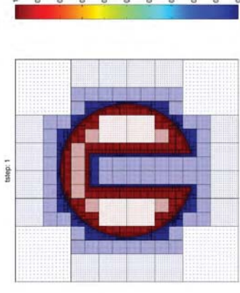
Abbildung 7: Ein Oktalbaum, welcher zur räumlichen Auflösung einer Zalesak-Scheibe erzeugt wurde
