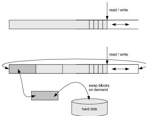
Abbildung 1. Der normale Stack (oben) wird durch ein Ringpufferkonzept mit nachgelagertem persistentem Medium abgelöst (unten).
