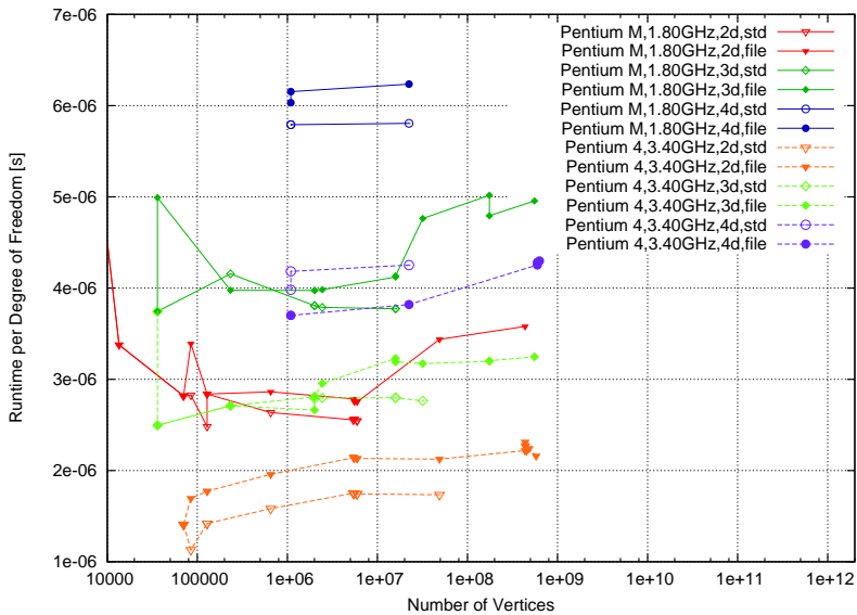
Abbildung 2: Rechenzeit pro Freiheitsgrad pro V-(1/0)-Zyklus. Der Dreitupel der Legende gibt Rechnertyp, Dimensionalität des Problems und verwendete Stack-Implementierung (Standard-C++-Klasse oder Datei-Ringpuffer-Konzept) an.
